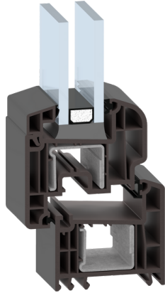
LINEA DESIGN (ANTA ARROTONDATA E FERMAVETRO INCLINATO)
