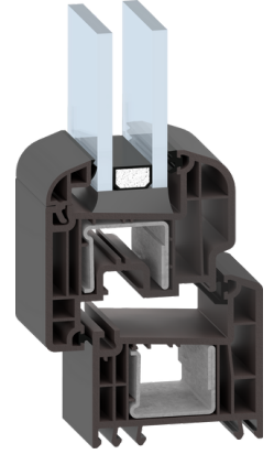
LINEA ROUND (ANTA ARROTONDATA E FERMAVETRO ARROTONDATO)
